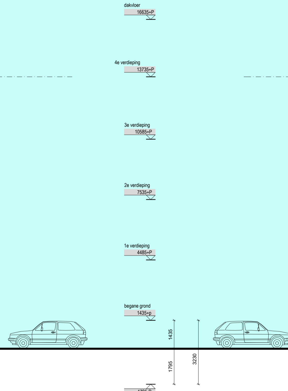
Noord-Westgevel
